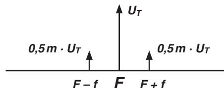
Abb. 1: Spektrumsamplituden und -frequenzen bei AM (m = 50%)
