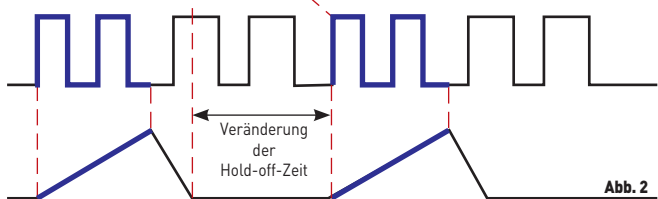
Abb. 1 zeigt das Schirmbild bei minimaler HOLD-OFF-Zeit (Grundstellung). Da verschiedene Teile des Kurvenzuges angezeigt werden, wird kein stehendes Bild dargestellt (Doppelschreiben).
